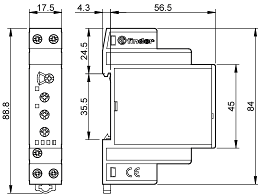
Тип 70.41 Винтовой клеммы
