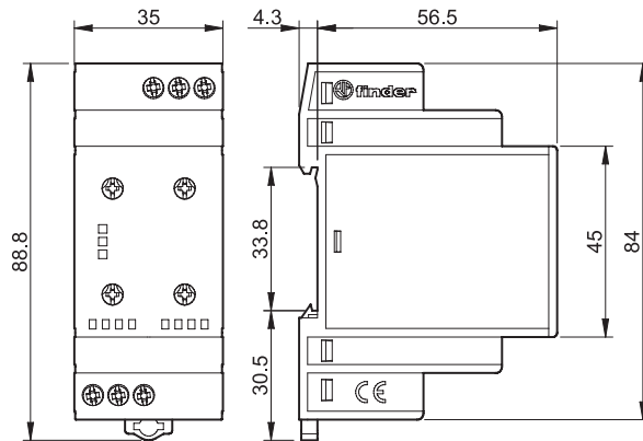
Тип 70.42 Винтовой клеммы
